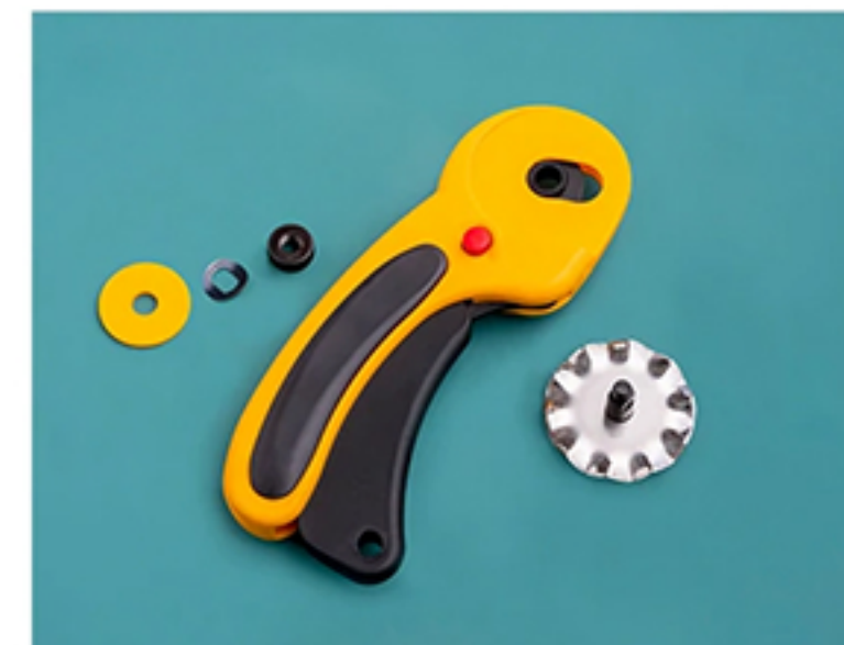
Nasuń na trzpień ostrze kształtowe
