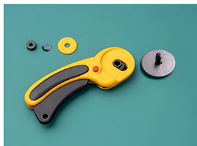
Zdejmij uchwyt z trzpienia i odłóż go na bok
