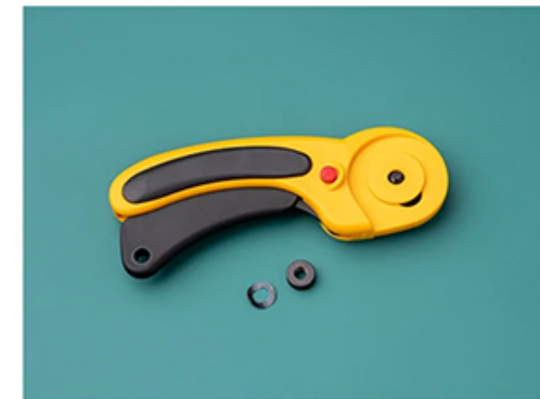
Zdejmij metalową podkładkę nie zmieniając pozycji, w jakiej była zamontowana
