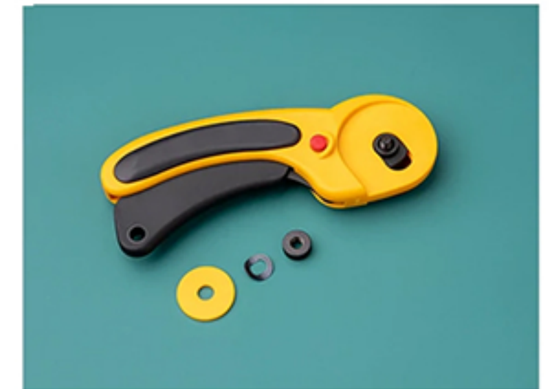
Zdejmij plastikową podkładkę
