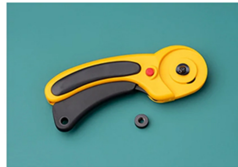
Odkręć nakrętkę i odłóż na bok nie zmieniając pozycji, w jakiej była zamontowana
